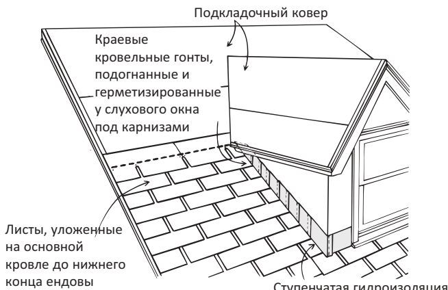
Рис. 6-4: Гидроизоляция фронтальной/боковой стены.
