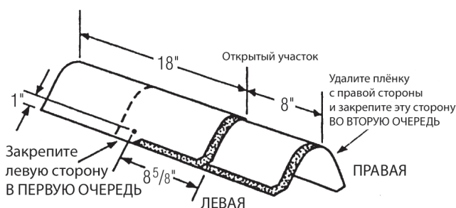
Рис. 16-19. Монтаж гонга Shangle® Ridge на рёбра и коньки.
