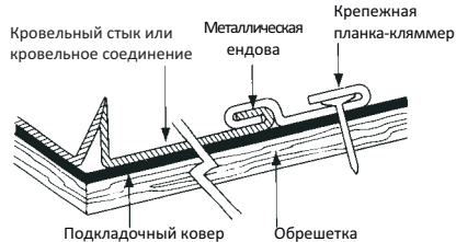
Рис. 6-21: Крепление металлической ендовы металлическими крепежными планками (кляммерами).
