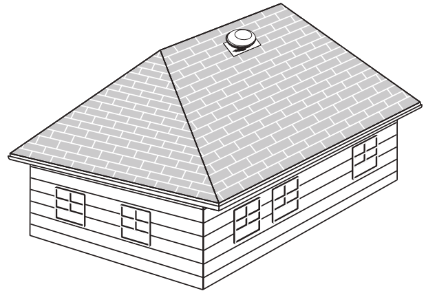
Рис. 7-25. Электрические вентиляторы служат для перемещения большого количества воздуха и являются хорошим выбором для вальмовых крыш, вентиляция которых затруднена.
