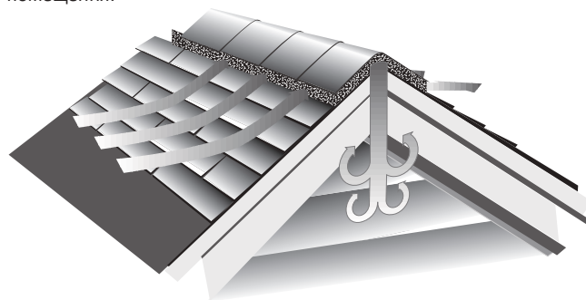
Рис. 7-22. Вентиляционный конёк с внутренней перегородкой или вообще без перегородки не «вытягивает» воздух из чердачного помещения через обе стороны вентиляционной секции.
