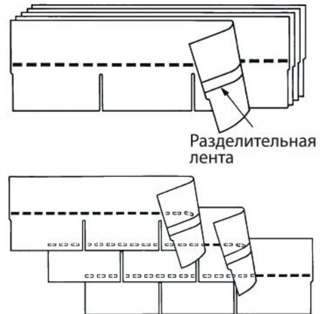
Рис. 2-2: Разделительная лента.
